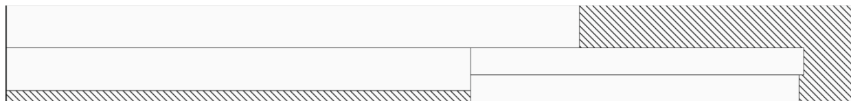
Рис. 2. Раскладка лекал на прикладном материале
